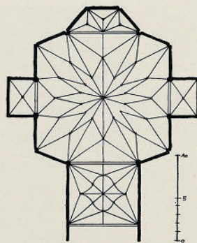
Abb. 14. Briviesca (Burgos). Sta. Clara. Grundriß.
