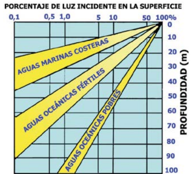
Figura 7. Reducción de la intensidad de la luz en aguas marinas (adaptado de Ros et al. , 1985; en Cognetti, 2001).
