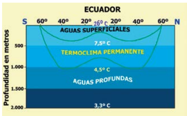
Figura 5. Sección esquemática de las principales capas térmicas de los océanos y de las temperaturas medias en el ecuador (Lalli y Parsons, 1997).
