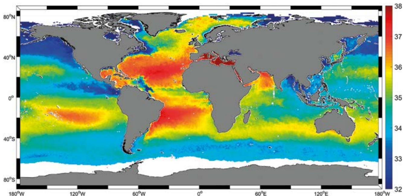
Figura 1. Salinidad en los océanos. Mapa promedio mensual de la salinidad de la superficie del océano para el mes de julio de 2015 (Reul et al. , 2020).
